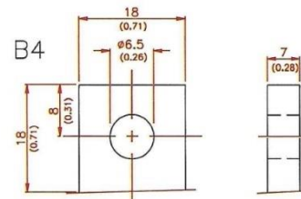
TAB Dimensions Max Torque 110 in-lb
